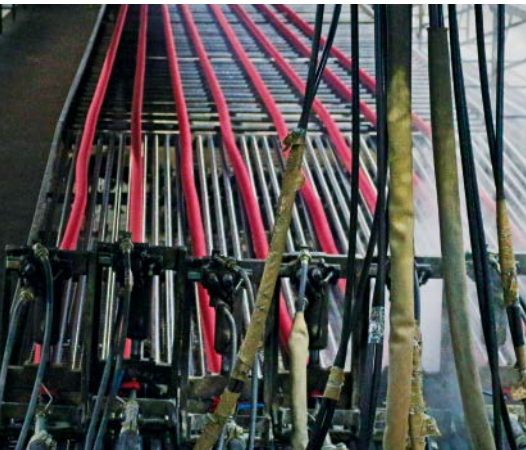
Vulkanisationsprozess auf 60 m langem Heiztisch
